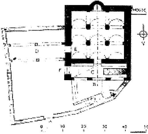
(تخطيط ٢٨) : مسجد بوفتاتة بسوسة فى شمال إفريقيا ٢٢٣ - ٢٢٦هـ / ٨٣٨ - ٨٤١م (التقسيم الثلاثى للمقدم). (عن : كريسيوزيل : الآثار الإسلامية الأولى ، ترجمة عبد الهادى عبلة ، دمشق ١٩٨٤م ، شكل ٥٥ ص ٣٥٣) .
